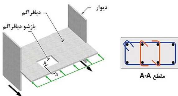
شکل ۲۴-۲۰ مثالی برای ضابطه ۳-۸-۲۰-۲
