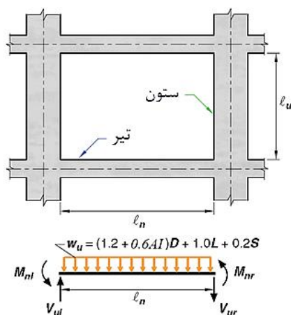
شکل ۲-۲۰ محاسبه برش در تیرها (روش مقاومتی)
