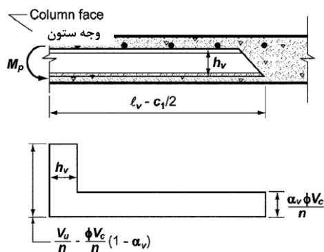
شکل ۸-۷ برش ایده‌آل در کلاهک برشی
