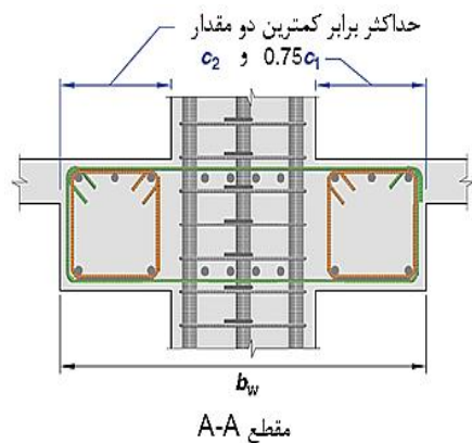
شکل ۵-۲۰ حداکثر عرض موثر در تیرهای پهن و آرماتور عرضی مورد نیاز
