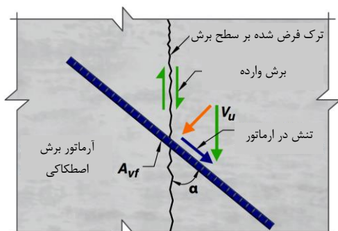
شکل ۸-۱۴-الف کشش در آرماتور برش اصطکاکی
