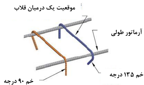
شکل ۱-۲۱ موقعیت قلاب‌های دوخت (سنگاقی)
