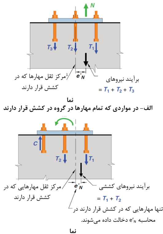
شکل ۱۸-۶ تعریف e'_N برای گروه مهار
