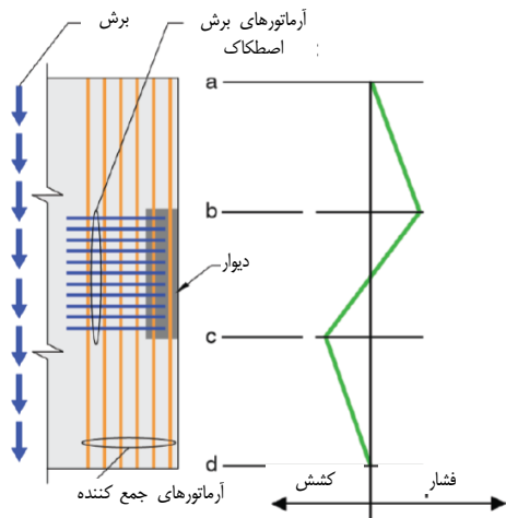
شکل ۷-۱۴ جمع‌کننده با عمق کامل و آرماتور مورد نیاز برای عملکرد برش اصطکاکی جهت انتقال نیروی جمع‌کننده به دیوار
