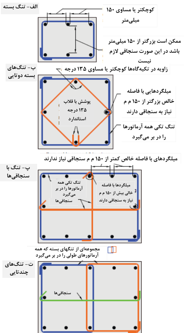
شکل ۱۶-۲۱ میلگردهای طولی دربر گرفته شده با خاموت‌ها و سنجاقی‌ها
