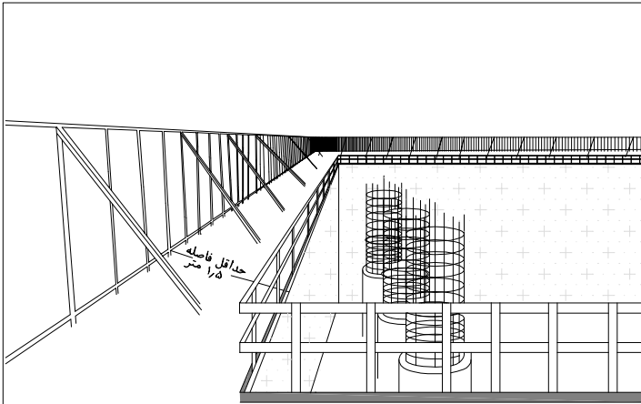
حصار حفاظتی موقت مطابق بند ۹-۵-۱۲
